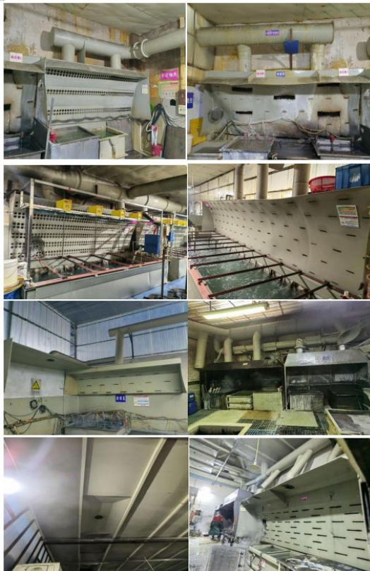
局部排风罩
